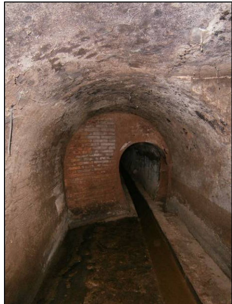
FOTO 28 – Detall del final de la galeria al costat de ponent del tram que discorre sota el carrer de Roger
