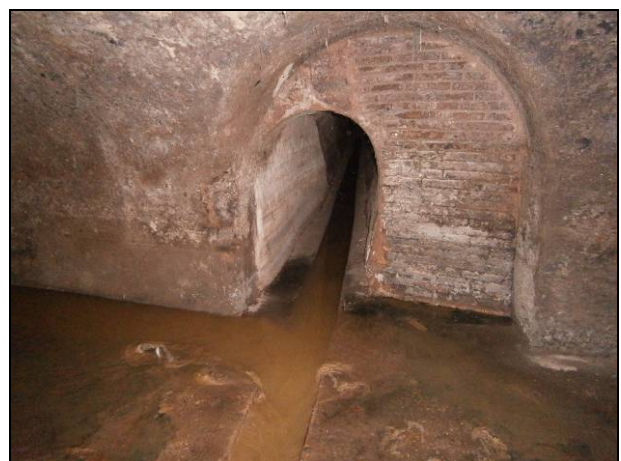
FOTO 24 - Clavaguera que entra pel costat de llevant del carrer de Roger
